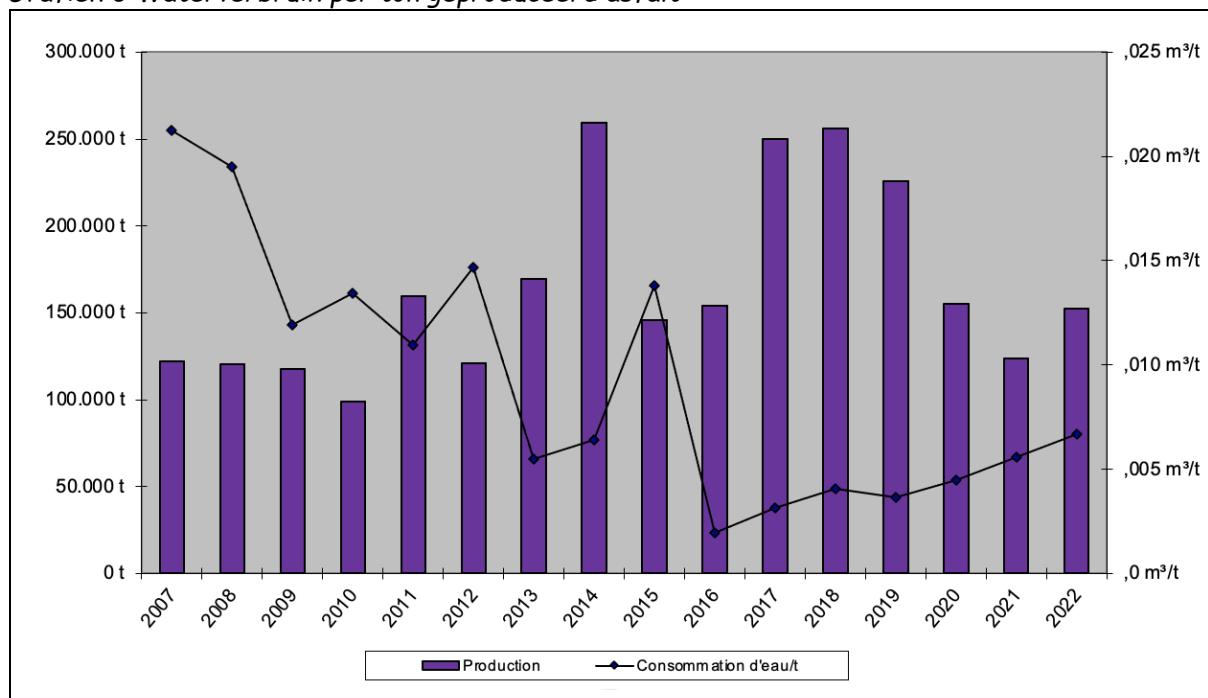
Grafiek 3 Waterverbruik per ton geproduceerd asfalt
