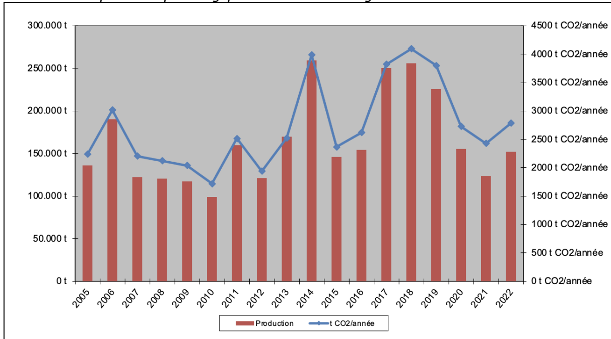
Grafiek 2 CO2-productie per ton geproduceerd asfaltmengsel
