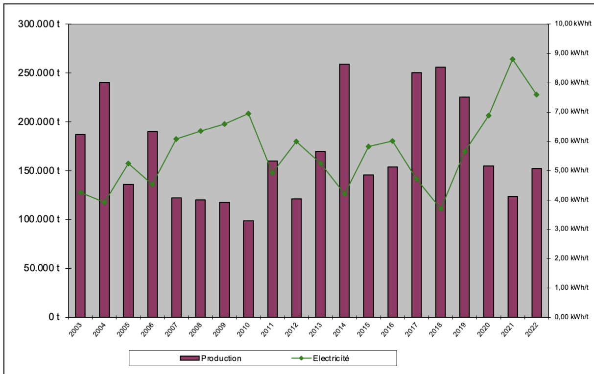
Grafiek 5 Elektriciteitsverbruik per ton geproduceerd asfaltmengsel
