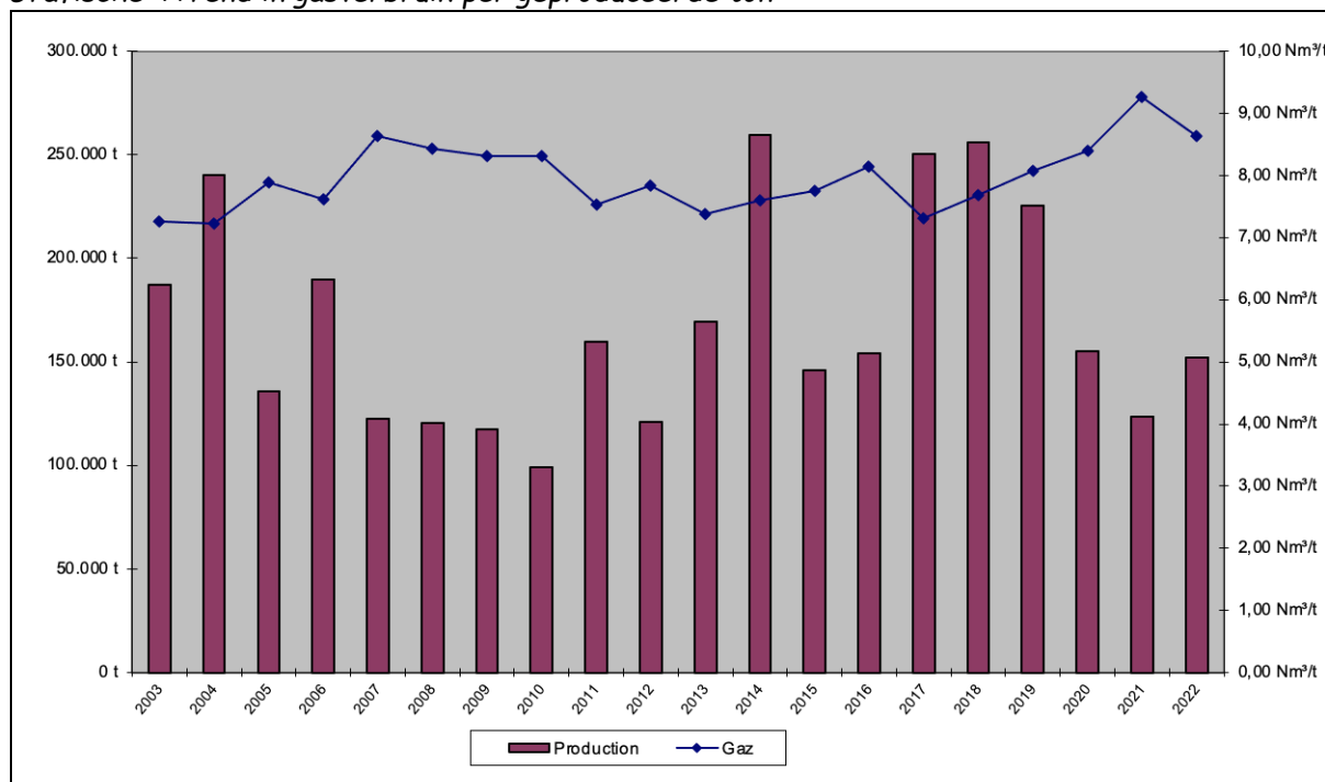
Grafische 4Trend in gasverbruik per geproduceerde ton
